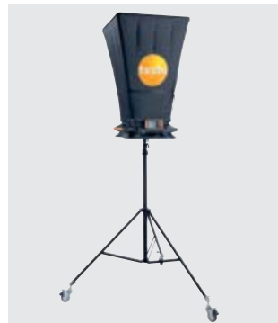
Standisches und rollbares Stativ mit zentraler Aufnahme für sicheres Arbeiten bei hohen Deckenauslässen.
