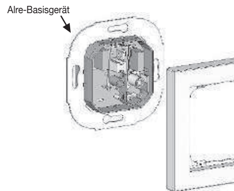
Alre-Unterputzgerät mit 55 x 55 mm Abdeckungset
