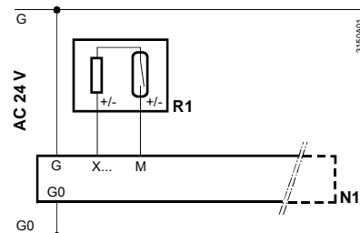
Schaltplan 5: Messteil mit Impulsgeber
